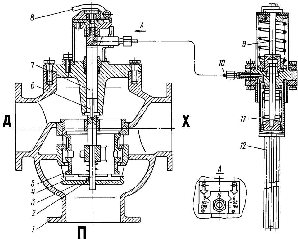
Конструкция терморегуляторов РТПД-125, РТПД-150
